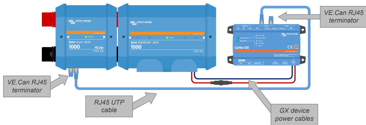
Esempio di cablaggio tra Lynx Shunt VE.Can e dispositivo GX
