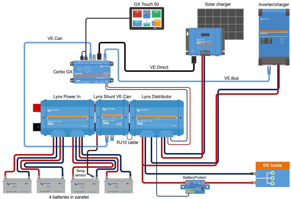
Sistema con Lynx Shunt VE.Can, batterie piombo acido e un Lynx Distributor
