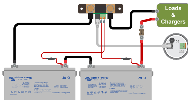
Monitor della batteria con monitoraggio ausiliare del punto medio.
