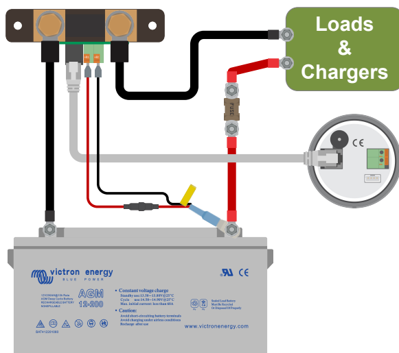
Monitor della batteria con rilevamento ausiliare della temperatura.
